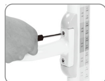
1. Установите ножкам и закрепите винтами
